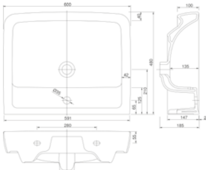
VIGCLE60 Umývadlo nábytkové 60 × 48 cm
