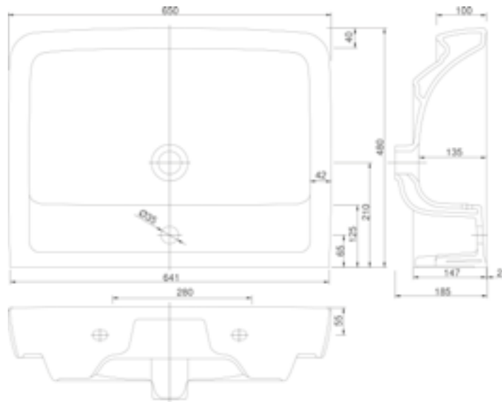
VIGCLE65 Umývadlo nábytkové 65 × 48 cm
