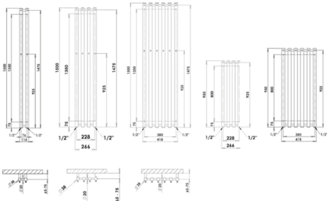
šírka 266 mm šírka 420 mm
