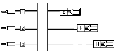
35. Sestava kabelu TT
