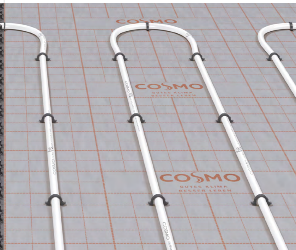
COSMO viacvrstvové potrubie s kyslíkovou bariérou PE-RT/AL/PE-RT 16x2 mm DIN CERTCO 3V379MVR
