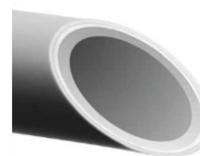
COSMO viacvrstvové potrubie s kyslíkovou bariérou PE-RT/AL/PE-RT 16x2 mm DIN CERTCO 3V379MVR
