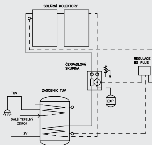
SCHÉMA PRO ZAPOJENÍ SAMOSTATNÝCH SOLÁRNÍCH SETŮ
